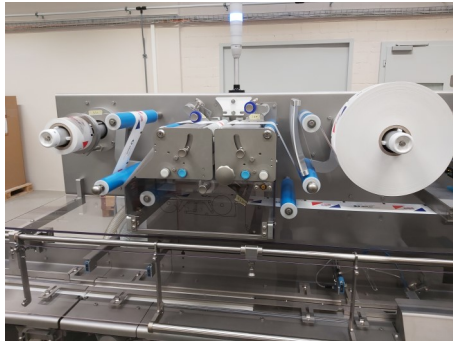
Automatischer Film-Spicer
